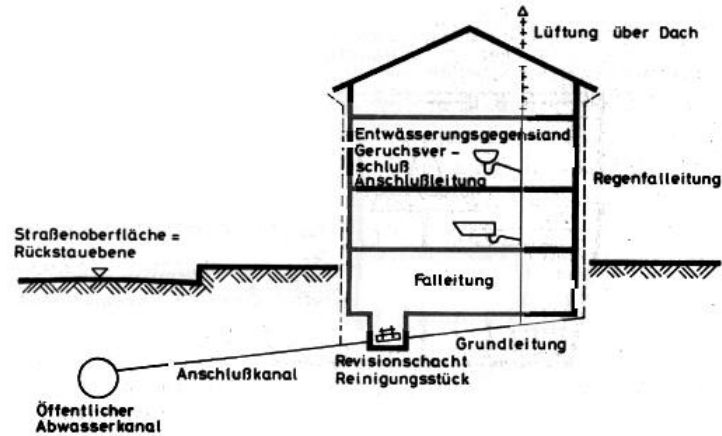
Schematische Darstellung einer Grundstücksentwässerung (Schnitt)
