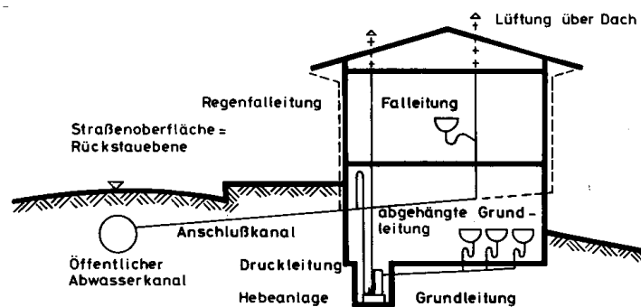
Schema für eine Hebeanlage in der Grundstücksentwässerung
